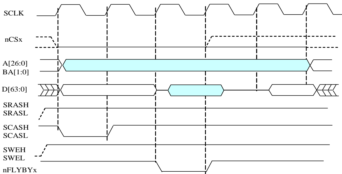
Рисунок 8.21. Передача одного слова данных из SDRAM в устройство ввода-вывода
