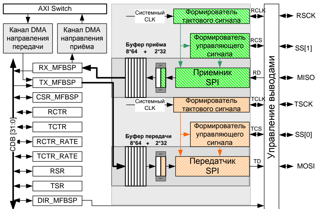
Рисунок 11.20. Структурная схема MFBSP для режима SPI
