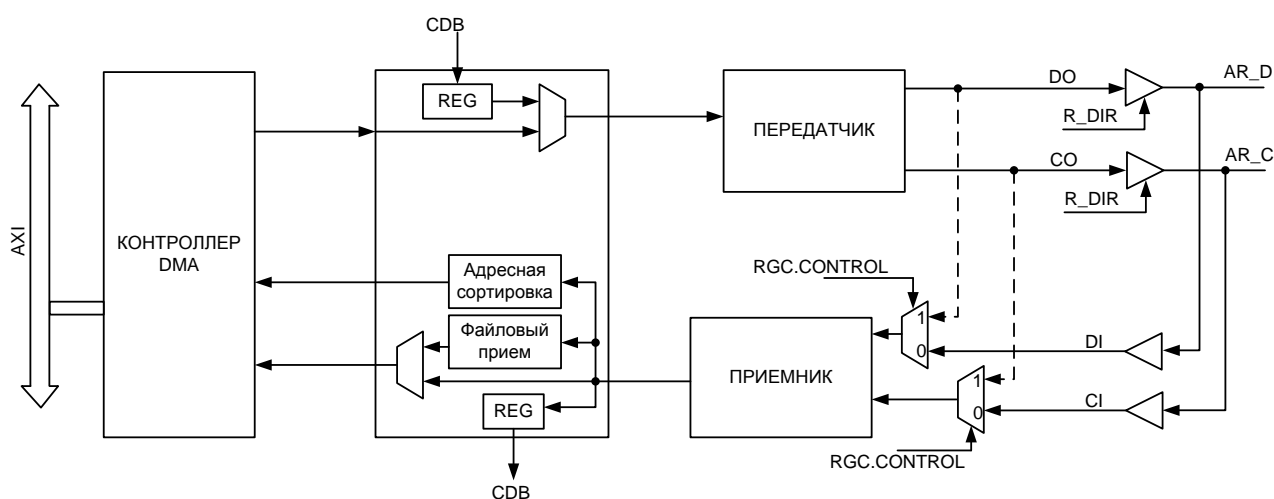
Рисунок 12.1. Структурная схема порта ARINC429
