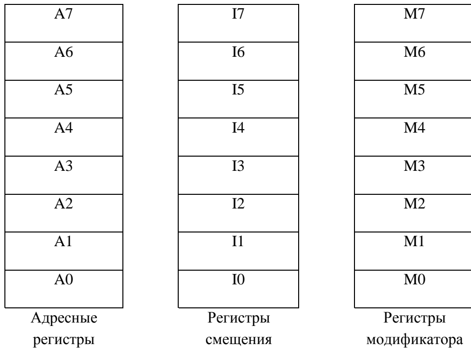
Рисунок 4.8. Программная модель AGU
