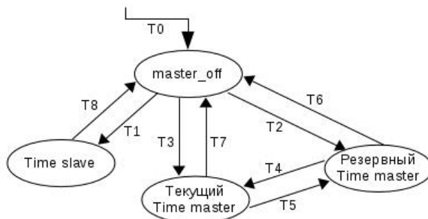
Рисунок 13.4. Диаграмма перехода состояний time master – time slave
