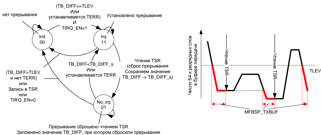
Рисунок 11.4. Механизм установки и сброса прерывания MFBSB_TXBUF. На рисунке TIRQ\_EN = (LEN \& LTRAN \parallel TEN \& SPI\_I2S\_EN)
