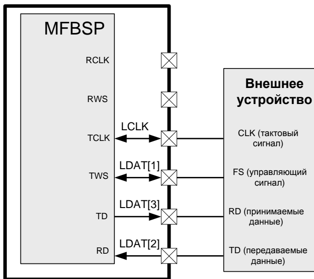
Рисунок 11.10. Соединение двух устройств по интерфейсу I2S в дуплексном режиме. Приёмник в зависимом от передатчика режиме (задействовано 4 внешних выводов). Как приёмником, так и передатчиком используются тактовый и управляющий сигналы с выводов TCLK и TWS. Направление выводов TCLK и TWS может быть произвольным в зависимости от требований внешнего устройства (режим №3 по Таблица 11.1)
