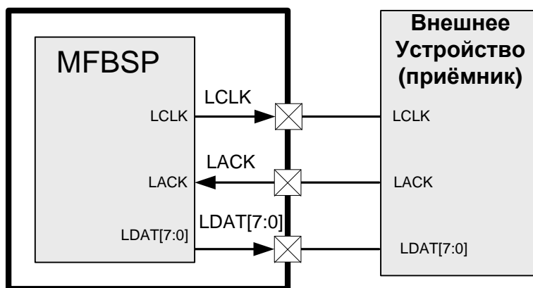
Рисунок 11.35. MFBSB в режиме передатчика LPORT (LCLK, LDAT-выходы, LACK - вход) (режим №2 по Таблица 11.1)
