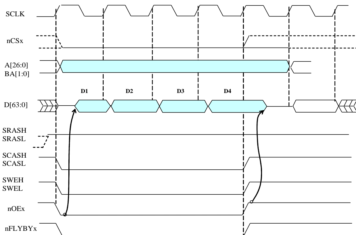
Рисунок 8.23. Передача 4-х слов данных из устройства ввода-вывода в SDRAM
