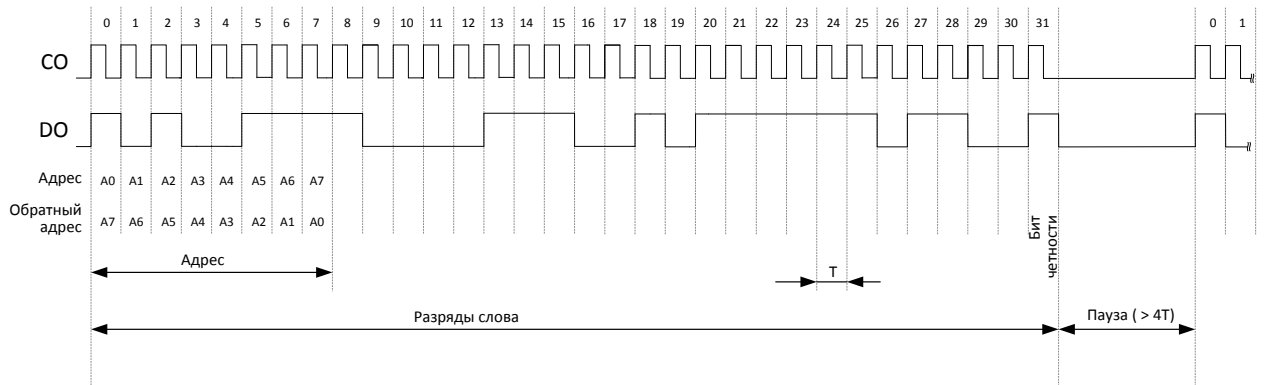
Рисунок 12.2. Передача одного слова (в режиме тактирующего сигнала на линии CO, R_CODE.CODE = 0)
