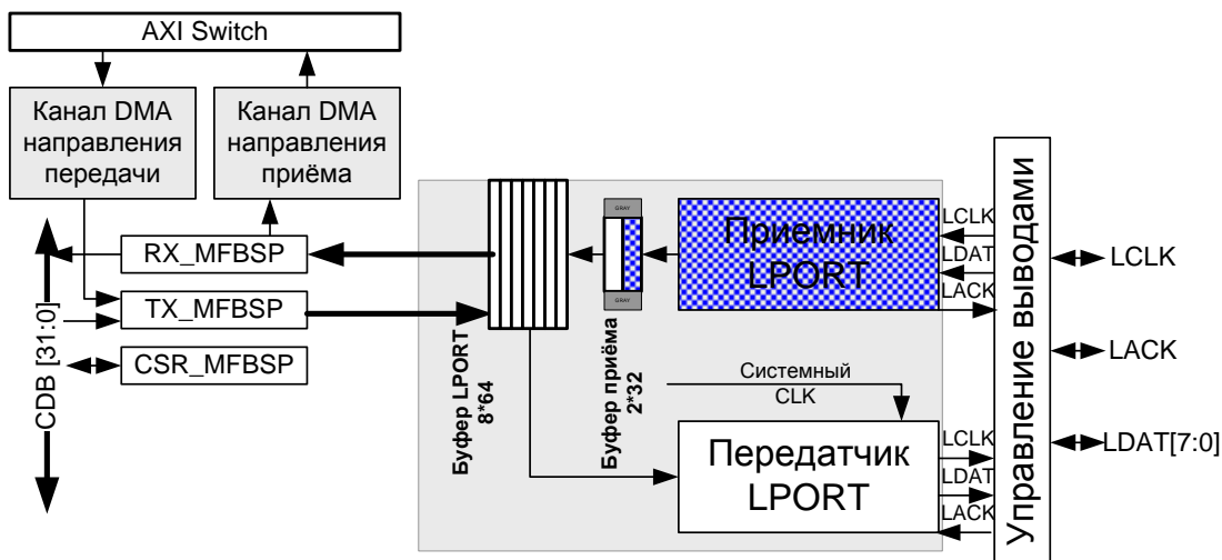
Рисунок 11.34. Структурная схема MFBSB для режима LPORT.
