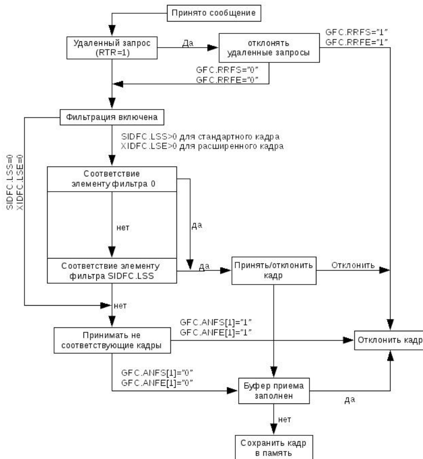
Рисунок 13.3. Схема фильтрации входящих сообщений
