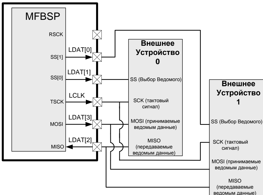
Рисунок 11.21. Подключение к MFBSIP двух ведомых устройств по интерфейсу SPI. Приёмник в зависимом от передатчика режиме (режим №6 по Таблица 11.1)
