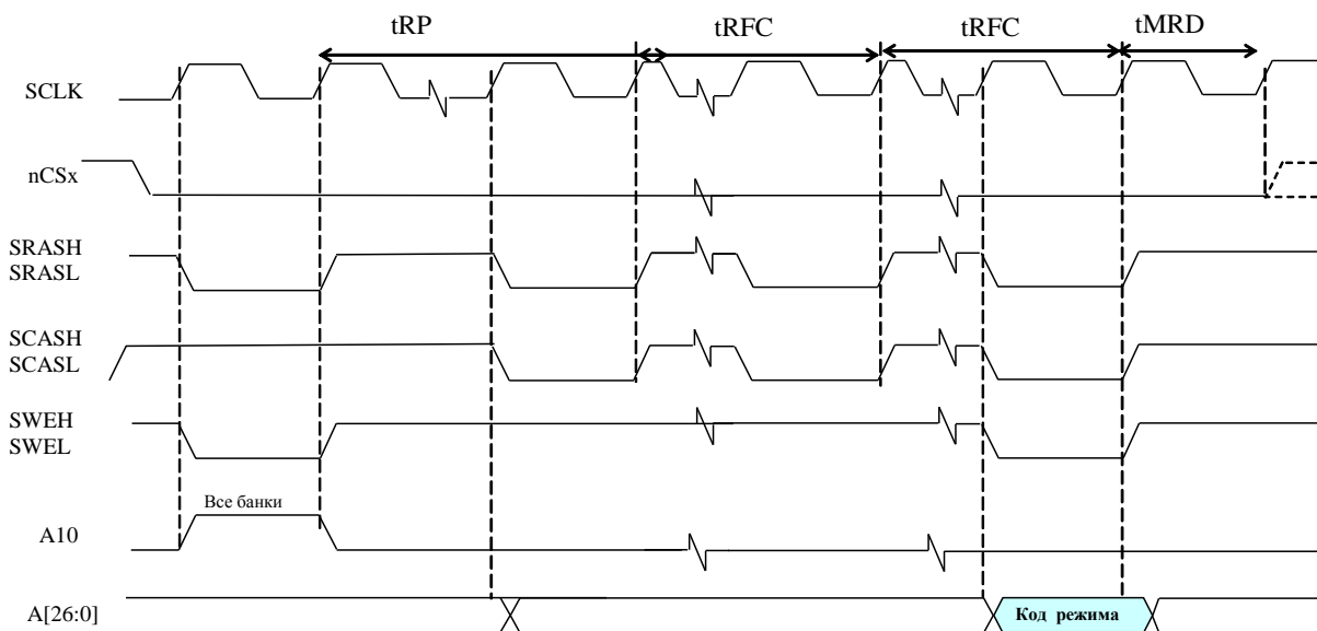
Рисунок 8.17. Инициализация SDRAM
