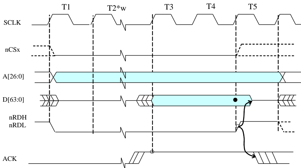
Рисунок 8.6. Чтение данных из асинхронной памяти с ожиданием сигнала АСК
