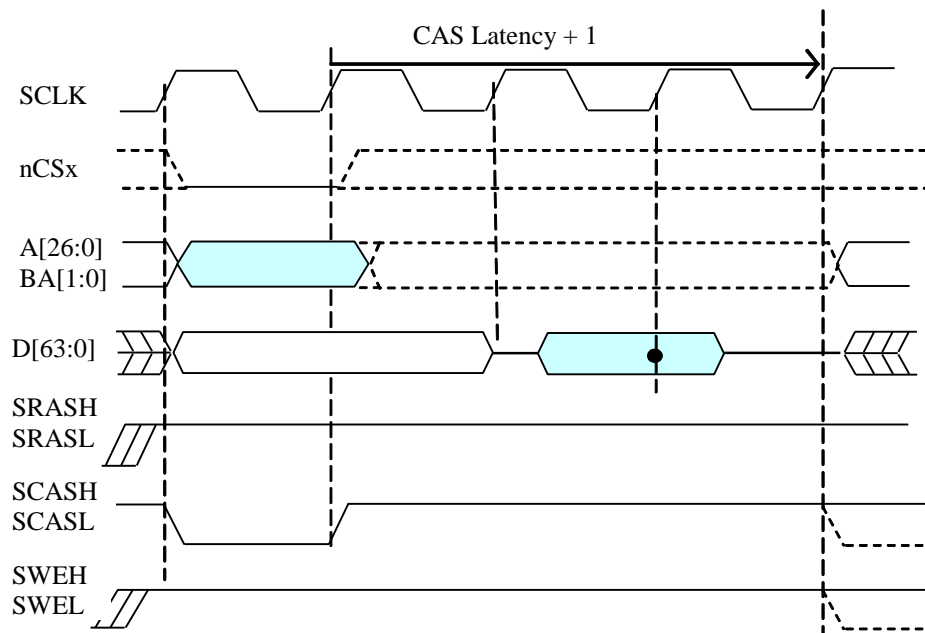
Рисунок 8.11. Чтение одного слова данных из SDRAM
