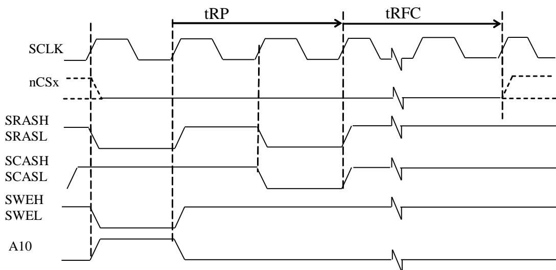
Рисунок 8.18. Регенерация SDRAM
