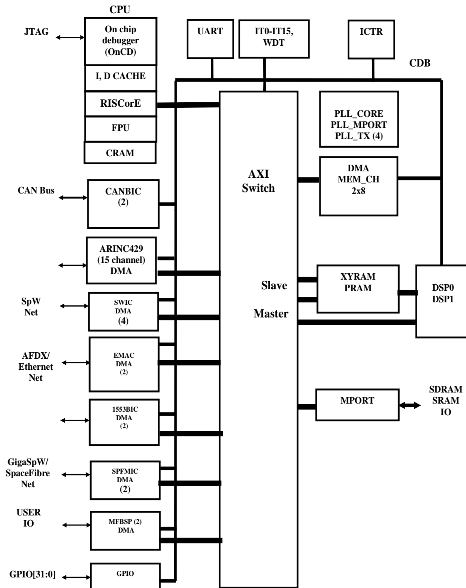
Рисунок 1.1. Структурная схема микросхемы 1892BM206
