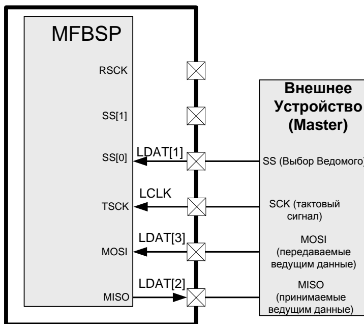
Рисунок 11.22. Подключение MFBSIP по интерфейсу SPI к внешнему ведущему устройству. Приёмник в зависимом от передатчика режиме (режим №6 по Таблица 11.1)
