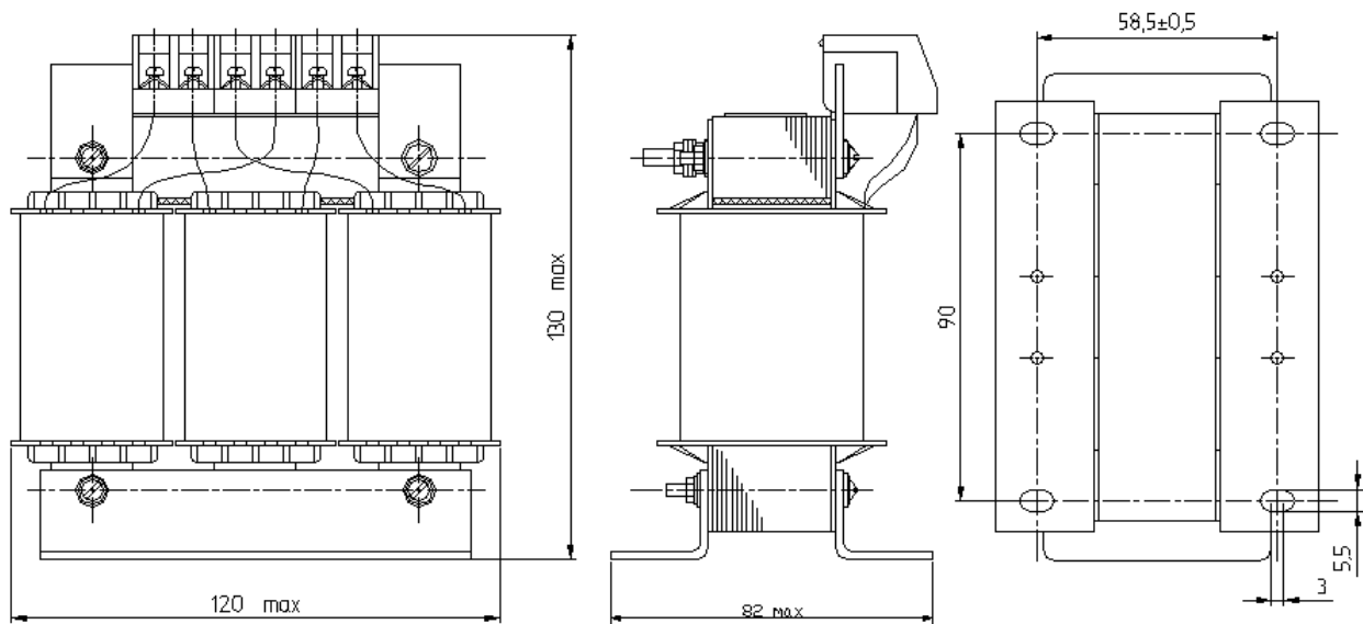
Рисунок 1- Общий вид DRT-2,2
